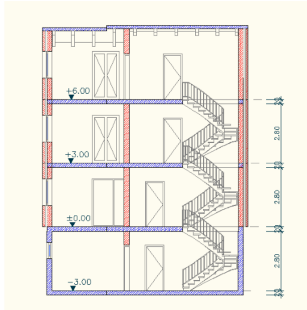
Abbildung 13: Beispielprojekt - Querschnitt Blickrichtung Norden
