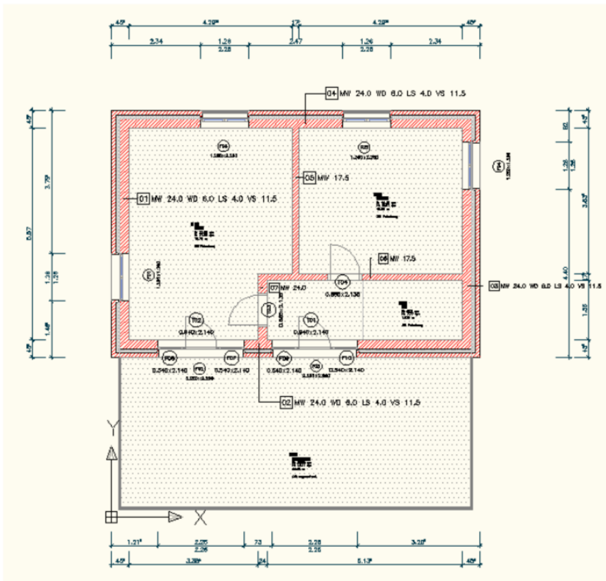
Abbildung 11: Beispielprojekt - Grundriss Dachgeschoss
