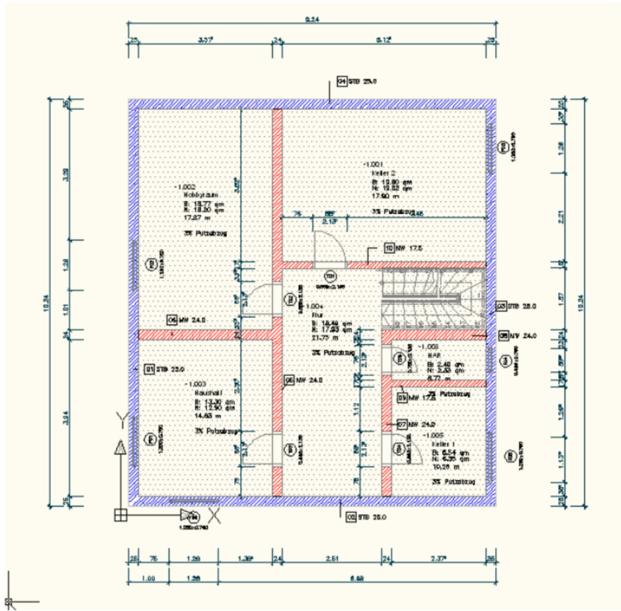
Abbildung 5: Beispielprojekt - Grundriss Kellergeschoss
