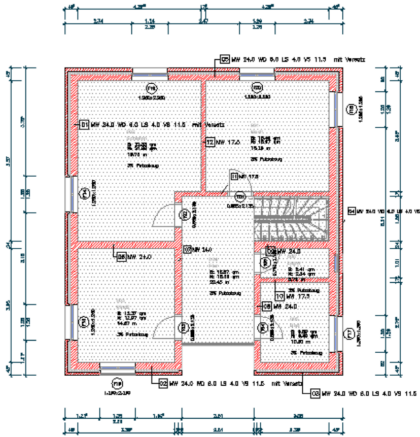
Abbildung 9: Beispielprojekt - Grundriss Obergeschoss
