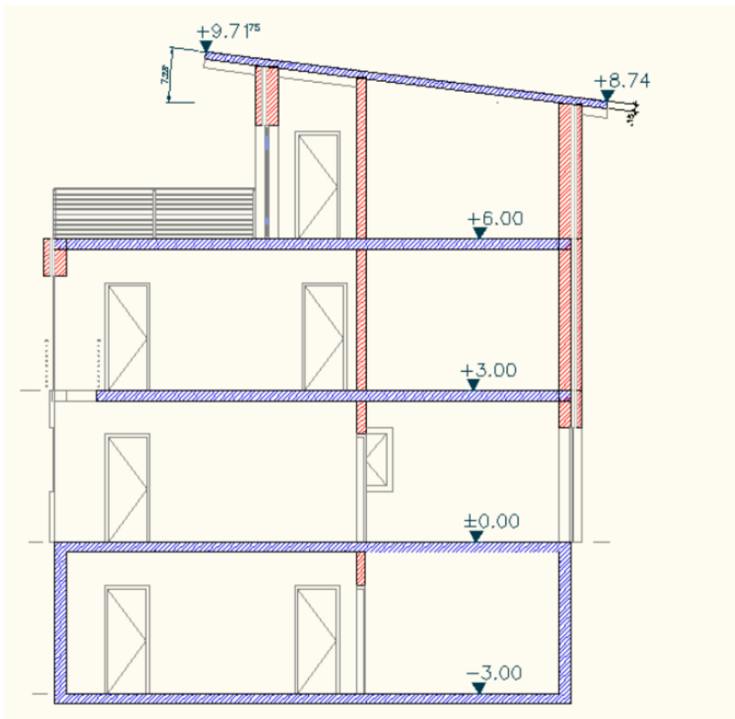
Abbildung 14: Beispielprojekt - Längsschnitt Blickrichtung Westen
