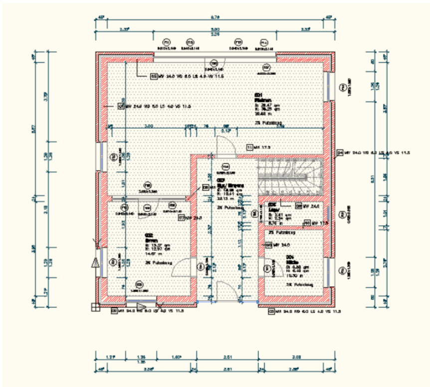
Abbildung 7: Beispielprojekt - Grundriss Erdgeschoss
